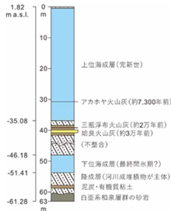
【小鳴門コア地質柱状図】
